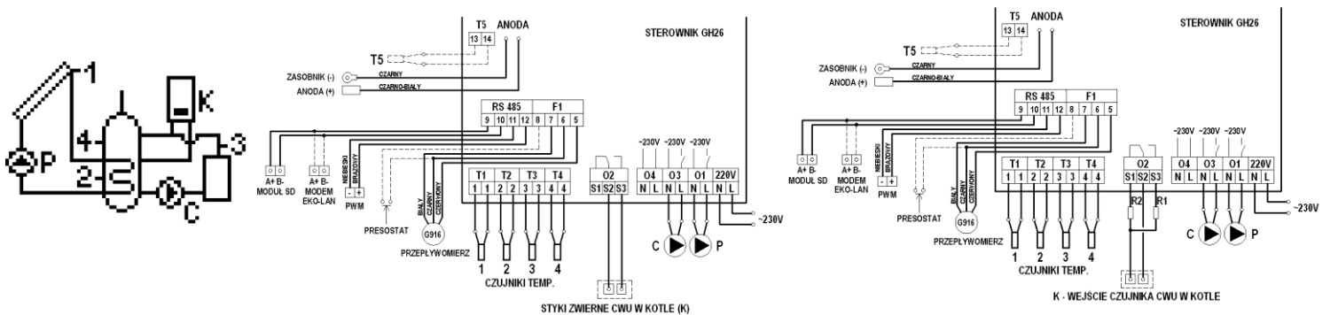
Rys. 16. Schemat ideowy oraz elektryczny instalacji układu nr 14.
