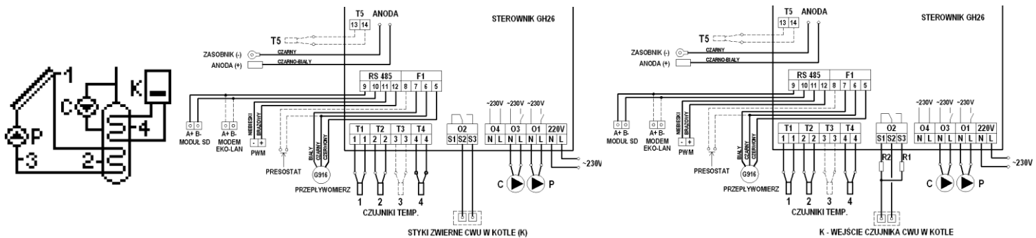
Rys. 5. Schemat ideowy oraz elektryczny instalacji nr 3.
