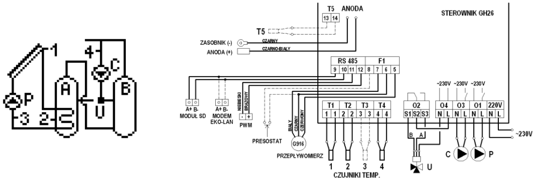
Rys. 10. Schemat ideowy oraz elektryczny instalacji układu nr 8.
