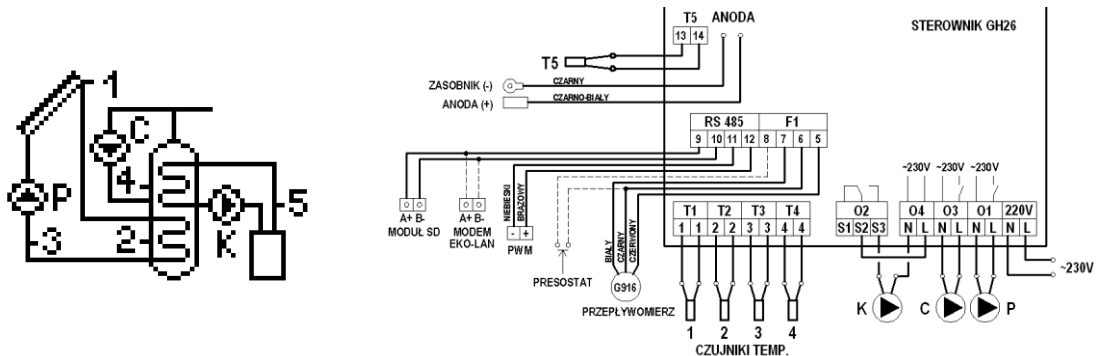
Rys. 8. Schemat ideowy oraz elektryczny instalacji nr 6.
