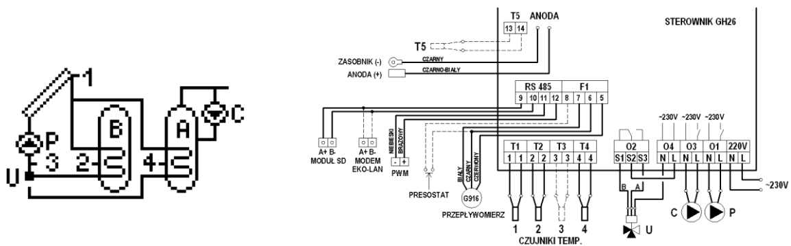
Rys. 13. Schemat ideowy oraz elektryczny instalacji układu nr 11.
