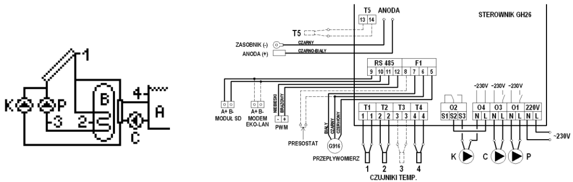
Rys. 12. Schemat ideowy oraz elektryczny instalacji nr 10.
