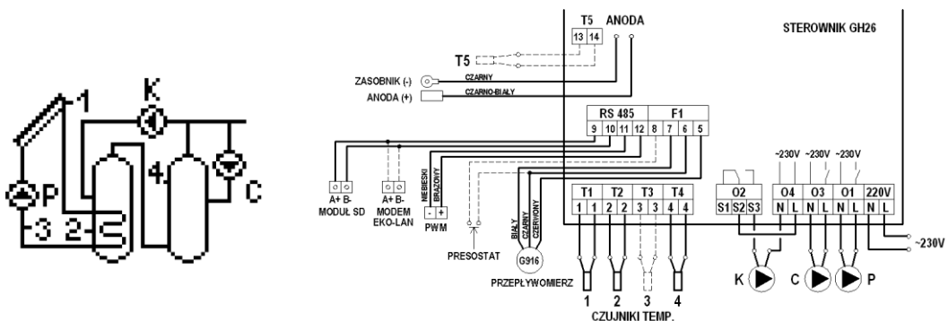
Rys. 9. Schemat ideowy oraz elektryczny instalacji nr 7.
