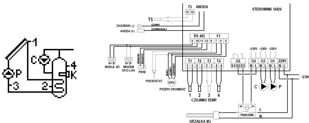
Rys. 6. Schemat ideowy oraz elektryczny instalacji nr 4.
