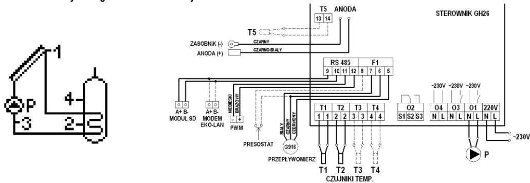
Rys. 3. Schemat ideowy oraz elektryczny instalacji nr 1.
