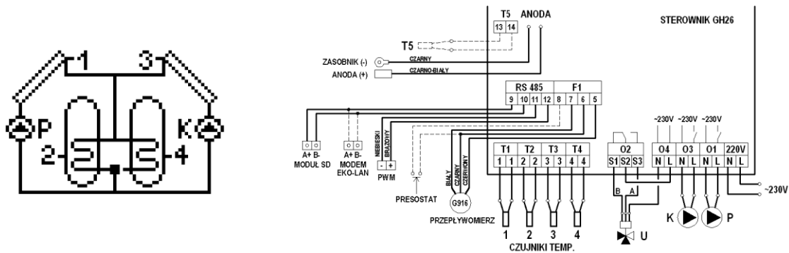
Rys. 18. Schemat ideowy oraz elektryczny instalacji układu nr 16.
