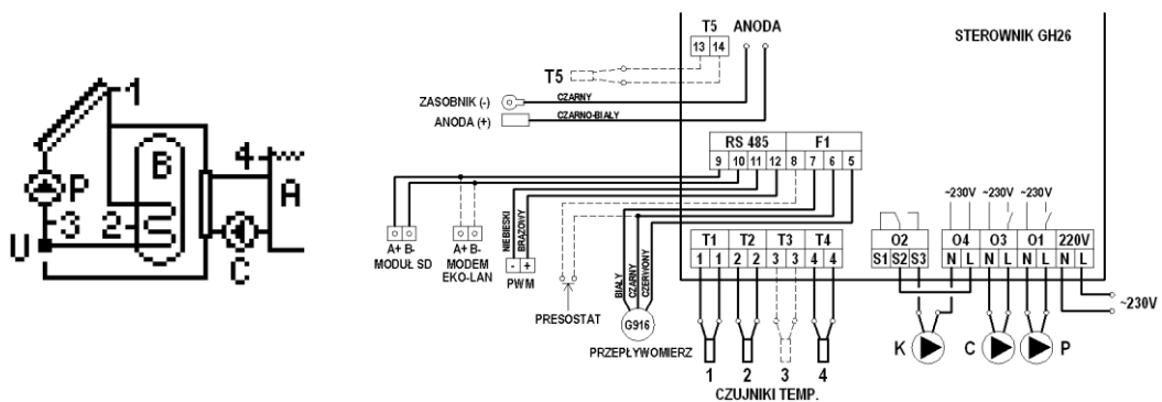
Rys. 11. Schemat ideowy oraz elektryczny instalacji nr 9.
