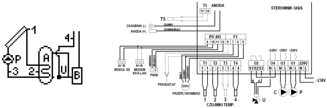
Rys. 15. Schemat ideowy oraz elektryczny instalacji układu nr 13.
