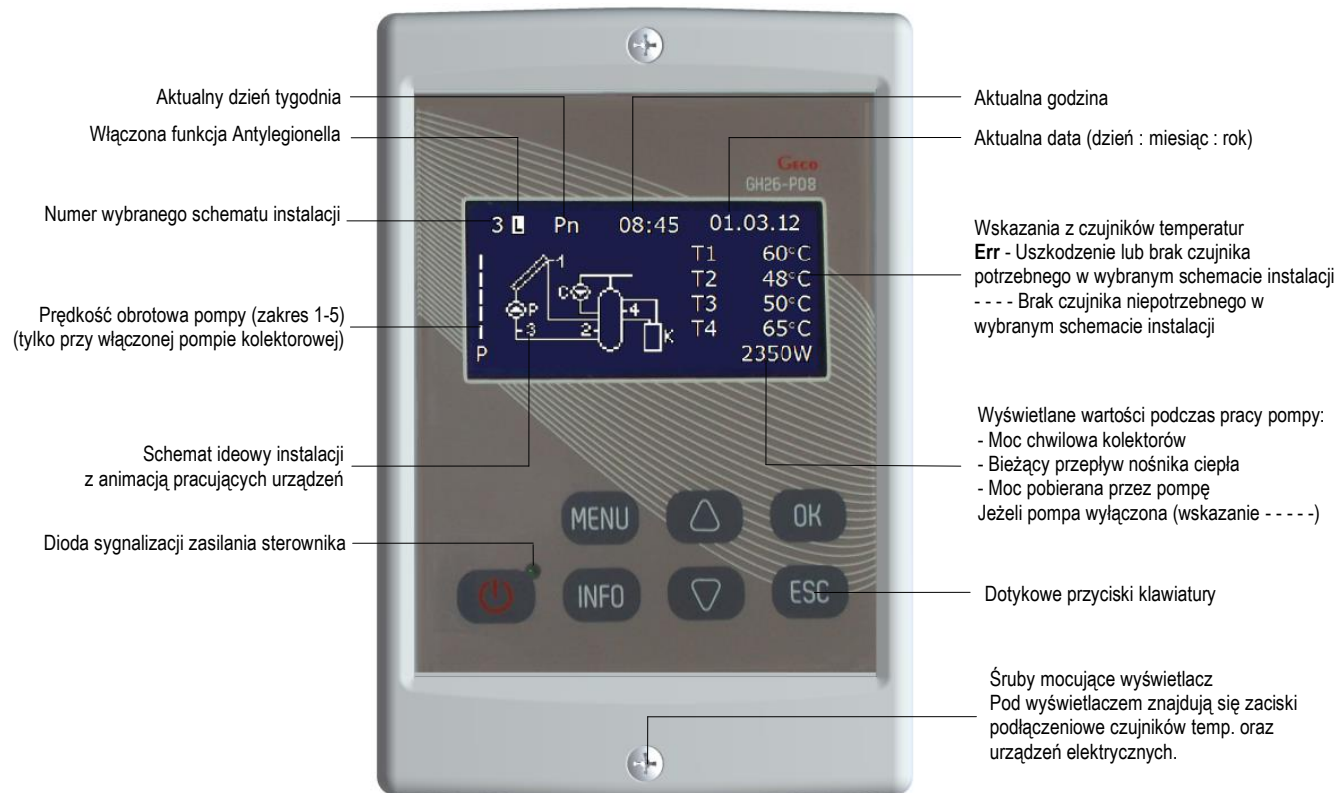
Rys. 2. Opis podstawowego ekranu na wyświetlaczu LCD
