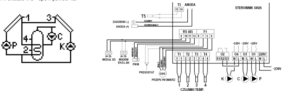
Rys. 17. Schemat ideowy oraz elektryczny instalacji układu nr 15.
