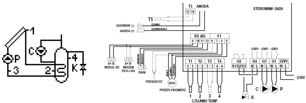
Rys. 19. Schemat ideowy oraz elektryczny instalacji układu nr 17.
