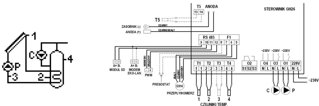
Rys. 4. Schemat ideowy oraz elektryczny instalacji nr 2.
