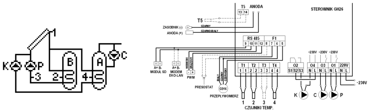
Rys. 14. Schemat ideowy oraz elektryczny instalacji układu nr 12.
