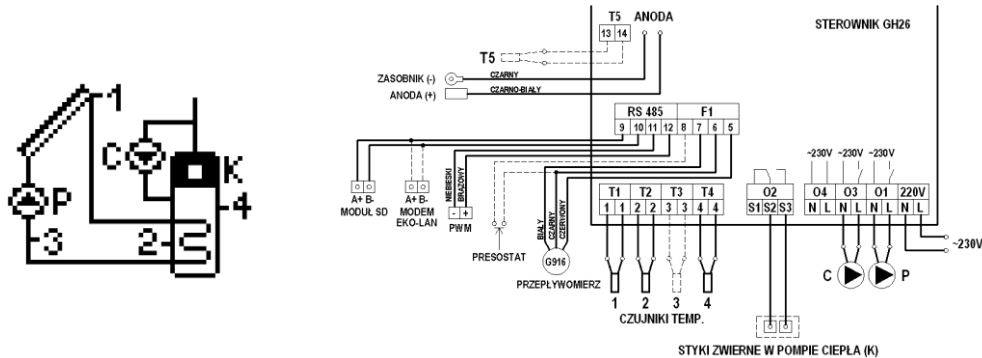
Rys. 7. Schemat ideowy oraz elektryczny instalacji nr 5.
