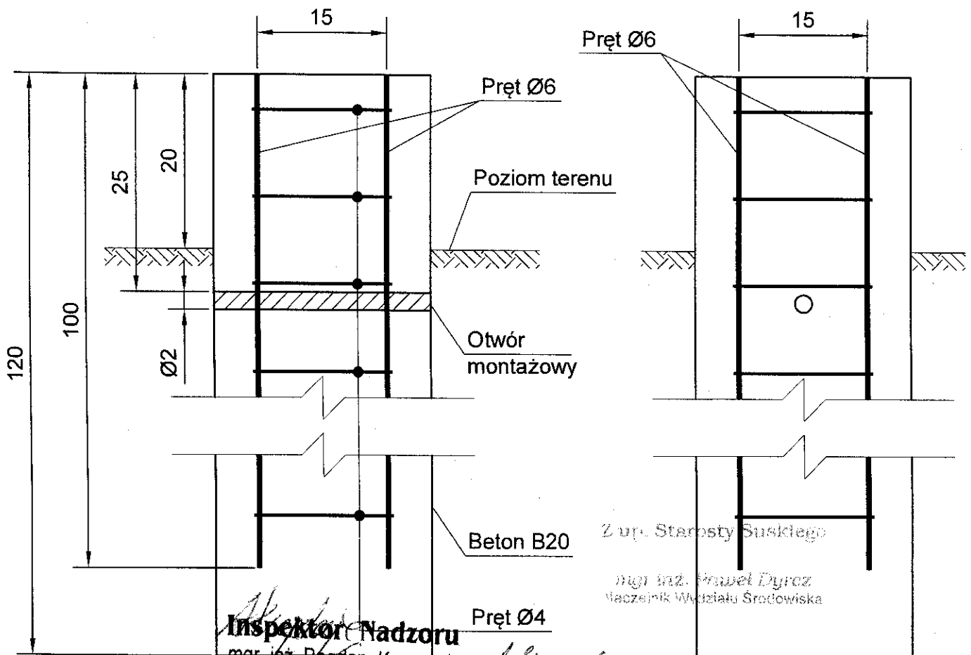
Przekrój B-B
