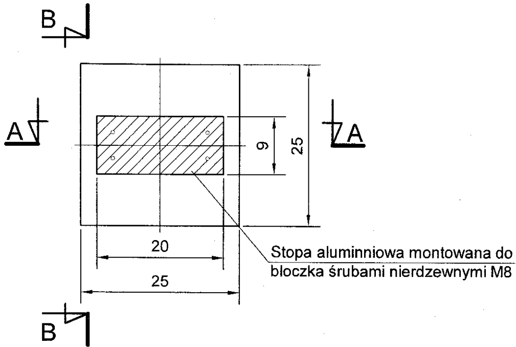
Przekrój A-A
